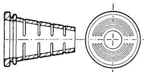
DOORVOERMOF MULTIFUNKTIONEEL
