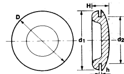
AFDICHTPLUG
